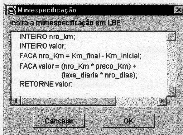
Figura 6 – Miniespecificação do Serviço CalcularTaxa da Classe Carro
