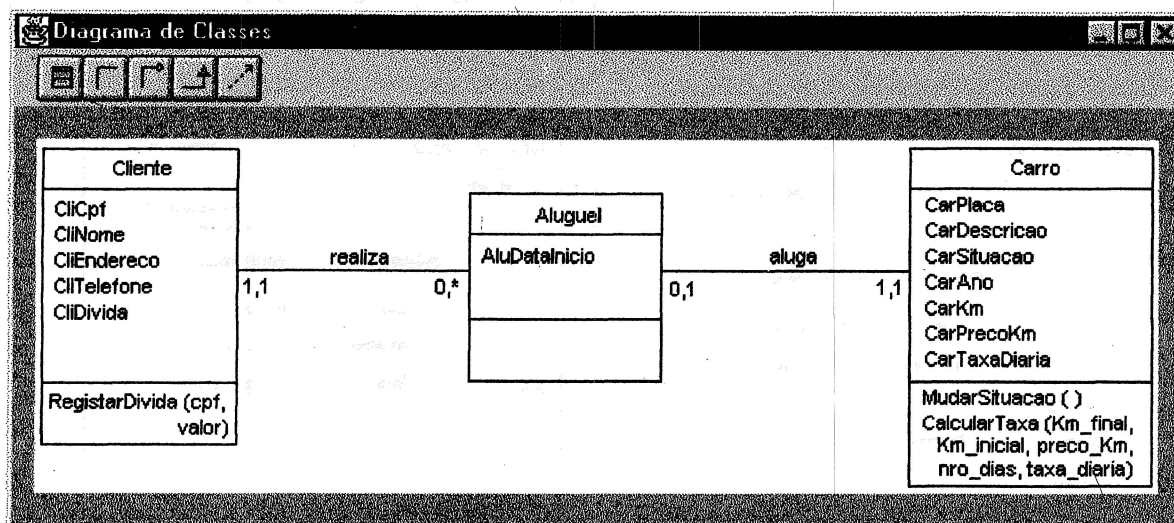
Figura 7 – Modelagem do Sistema de Locadora de Automóveis na JavaRC
