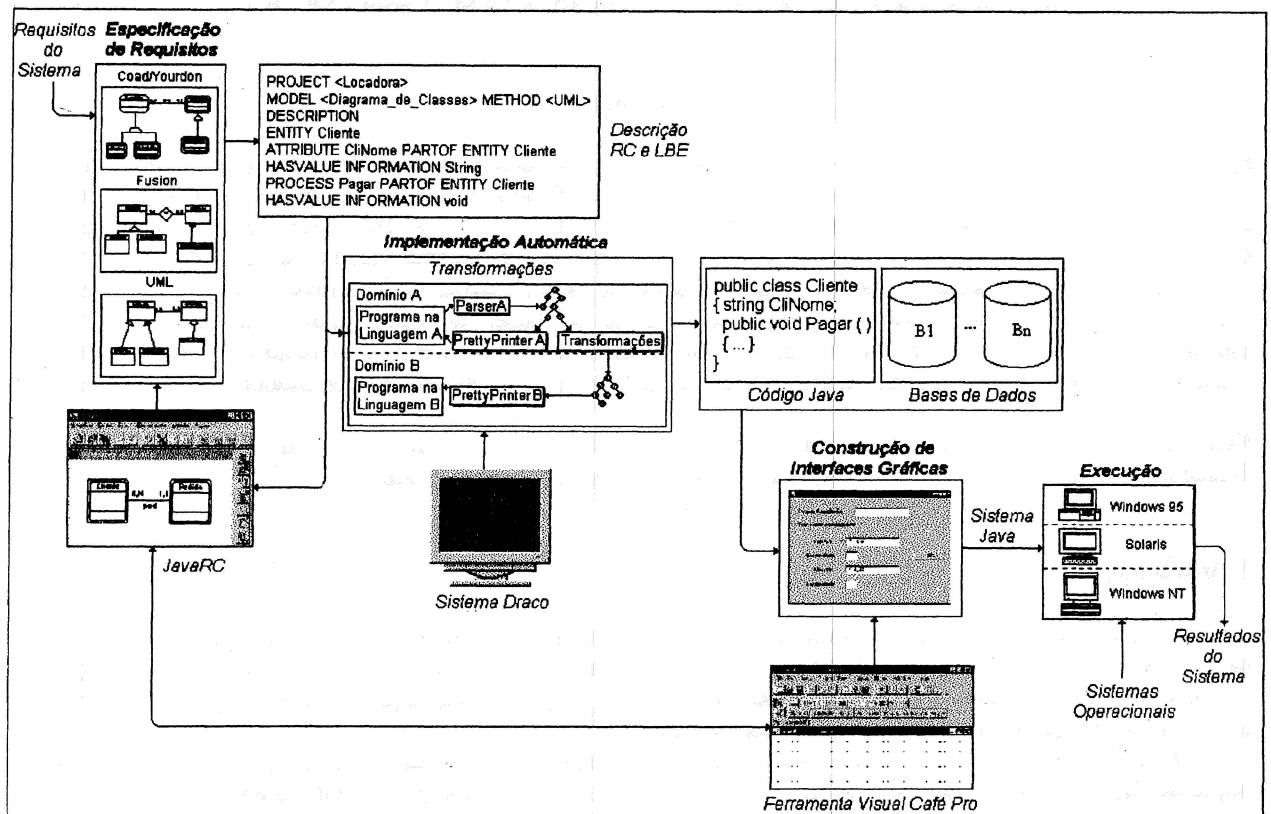
Figura 1 - Visão Geral da Ferramenta JMVCase
