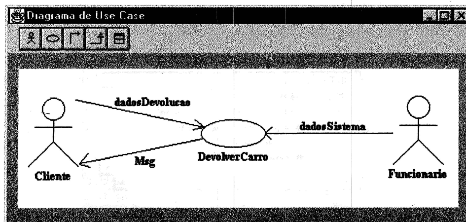
Figura 8 – Modelagem do Diagrama de UseCase para a Atividade DevolverCarro
