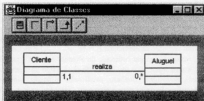
Figura 2 - Interface da ferramenta JavaRC para Modelagem de um Sistema
